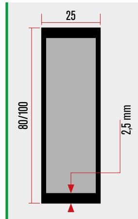
Profili a sezione rinforzata 2,5 mm. Sides with 2.5 mm reinforced section.
